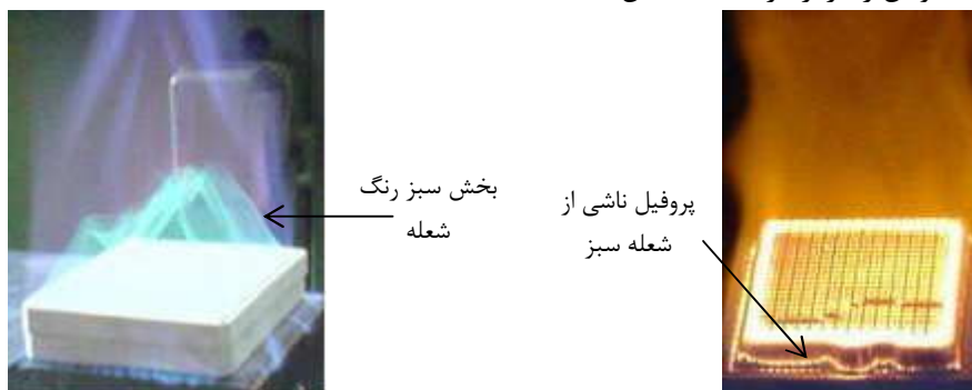
شکل 7- نفوذ قسمت سبز رنگ شعله در سرامیک ها و شکستن آنها در اثر تنش حرارتی
