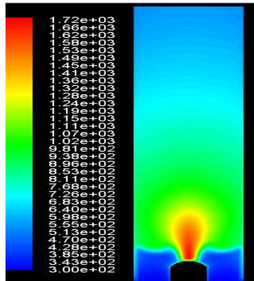
شکل 3 - توزیع دما در کوره T(K)
