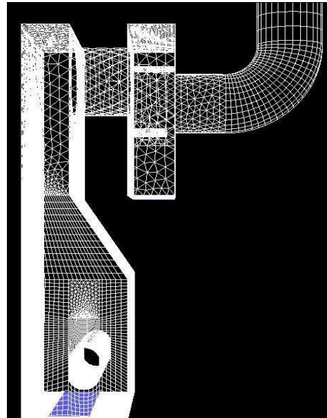
شکل 1- کوره کامل بخاری انتخابی
