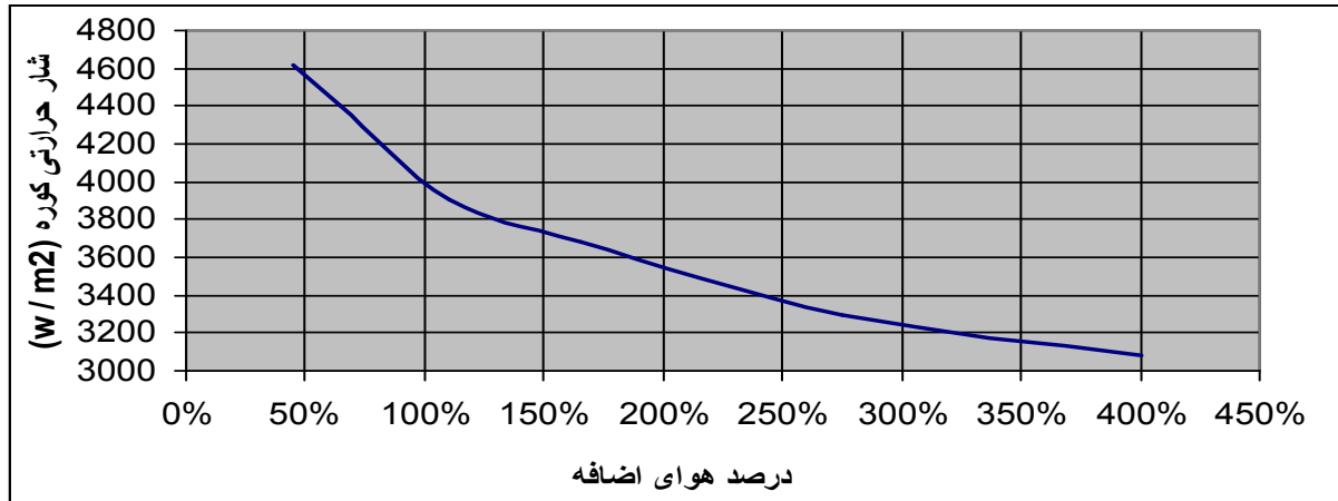
نمودار 1 - تاثیر هوای اضافه بر انتقال حرارت (بازده) بخاری به کمک نرم افزار
