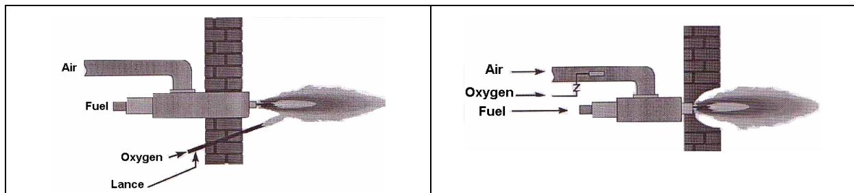
شکل ۲- (راست) شعله پیش مخلوط OEC - (چپ) لنس اکسیژن
