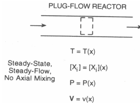
شکل ۱: شمای رآکتور پلاگ.
