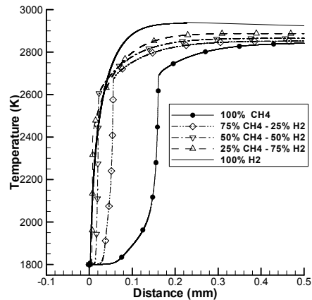
شکل (۴) - تغییرات دما در طول رآکتور در \phi = 1
