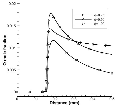
شکل (۱۵) - تغییرات کسر مولی O در طول رآکتور در f = 0
